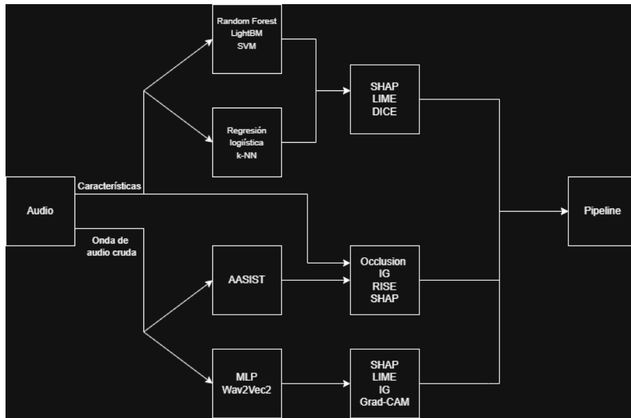
Figura 43: Arquitectura del pipeline.
